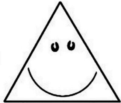
Triangolo
