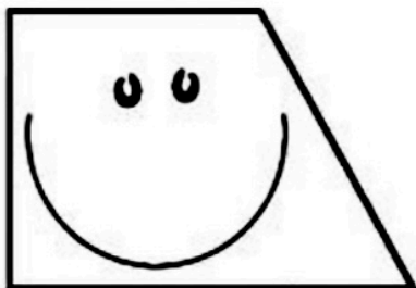
Trapezio
