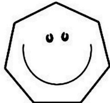
Ettagono
