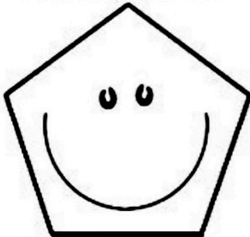
Pentagono
