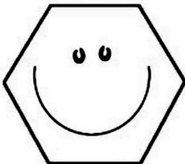
Esagono
