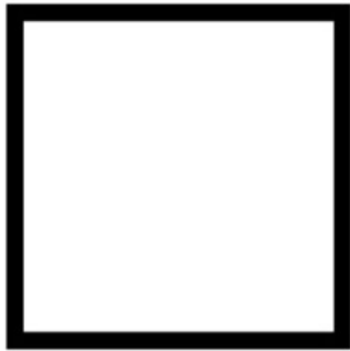
Linea orizzontale
