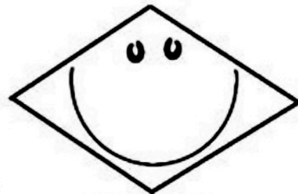
Rombo
